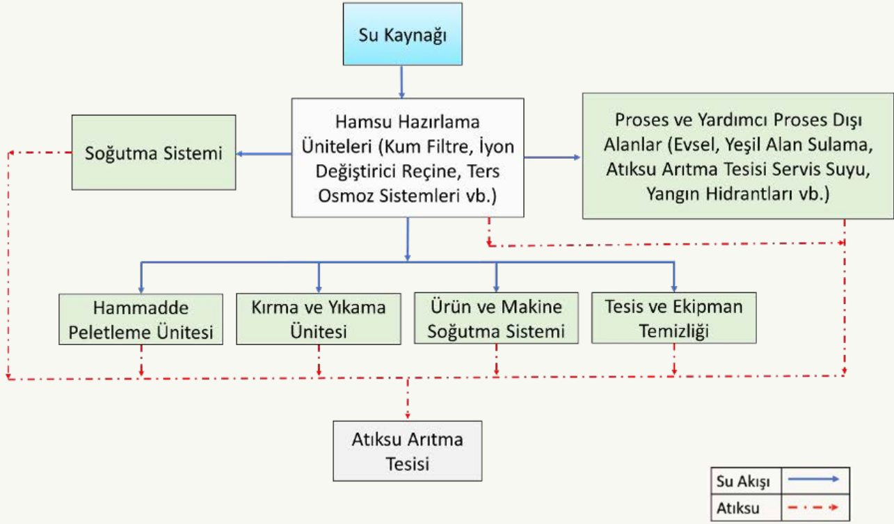
Tasnif Edilmiş Materyallerin Geri Kazanımı Sektörü Su Akım Şeması
