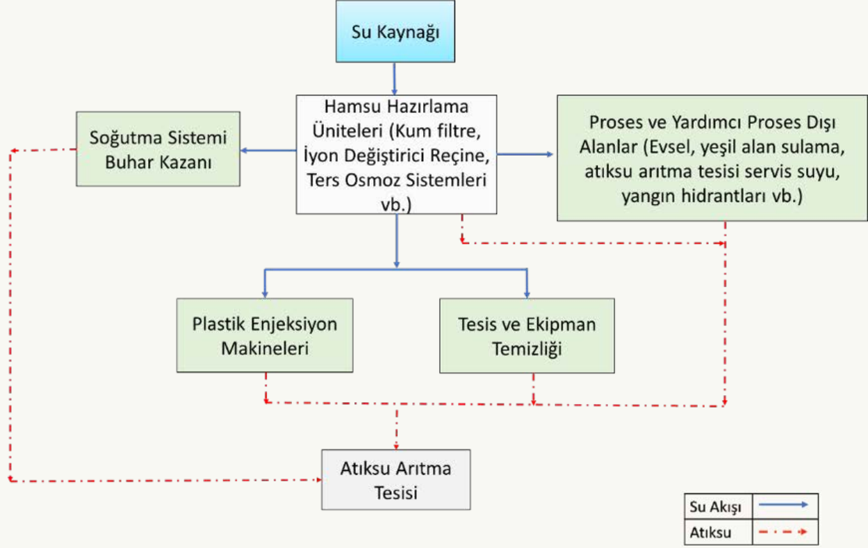
Oyun ve Oyuncak İmalatı Sektörü Su Akım Şeması
