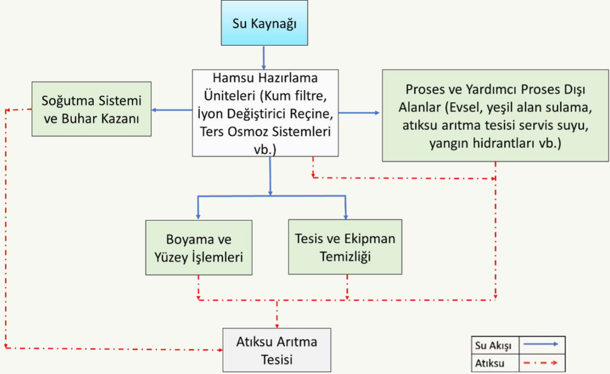
Gemilerin ve Yüzen Yapıların İnşası Sektörü Su Akım Şeması
