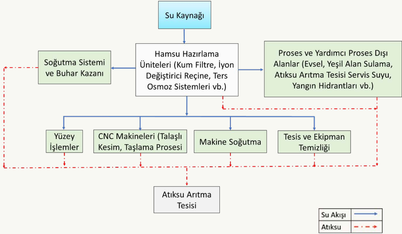
Rulman, Dişli/Dişli Takımı, Şanzıman ve Tahrik Elemanlarının İmalatı Sektörü Su Akım Şeması
