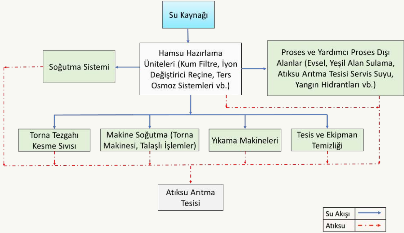
Akışkan Gücü İle Çalışan Ekipmanların İmalatı Sektörü Su Akım Şeması
