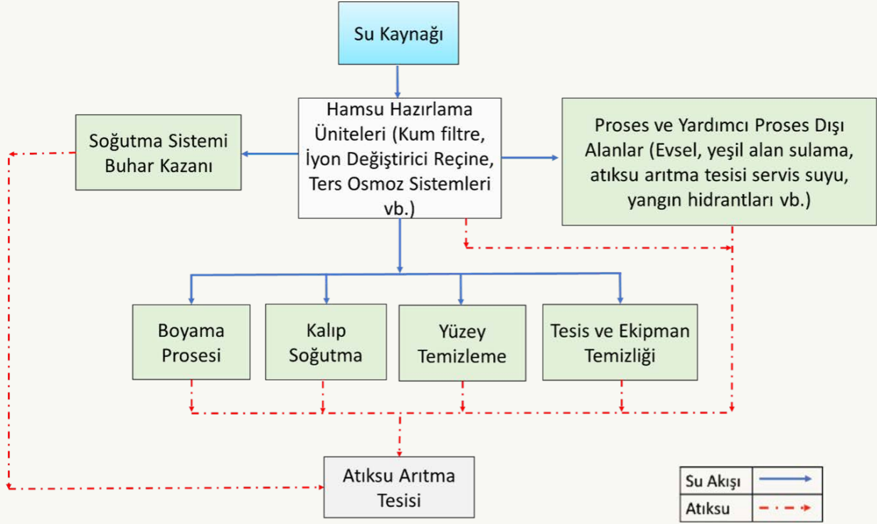
Tüketici Elektronik Ürünlerinin İmalatı Su Akım Şeması
