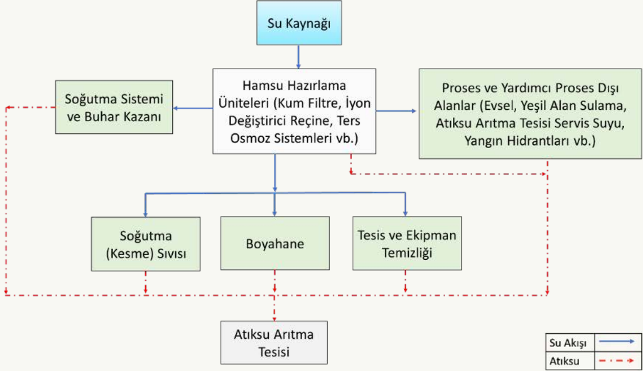
Metallerin Makinede İşlenmesi ve Şekil Verilmesi Sektörü Su Akım Şeması
