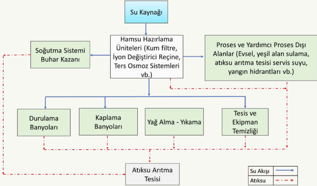
Metallerin İşlenmesi ve Kaplanması Sektörü Su Akım Şeması
