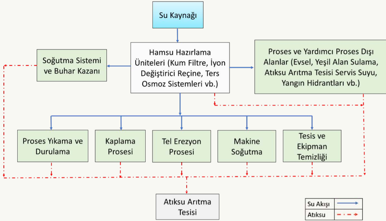
Metallerin Dövülmesi, Preslenmesi, Baskılanması ve Yuvarlanması; Toz Metalürjisi Sektörü Su Akım Şeması
