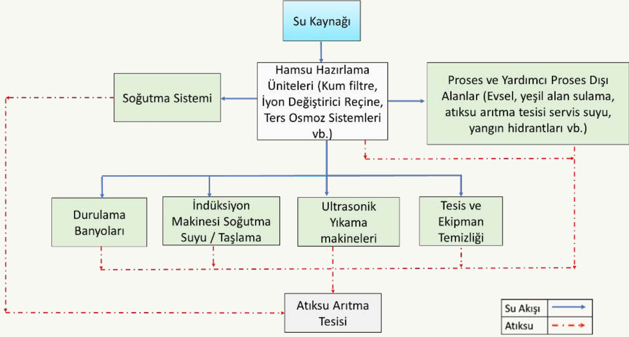
Çatal-Bıçak Takımları ve Diğer Kesici Aletlerin İmalatı Sektörü Su Akım Şeması
