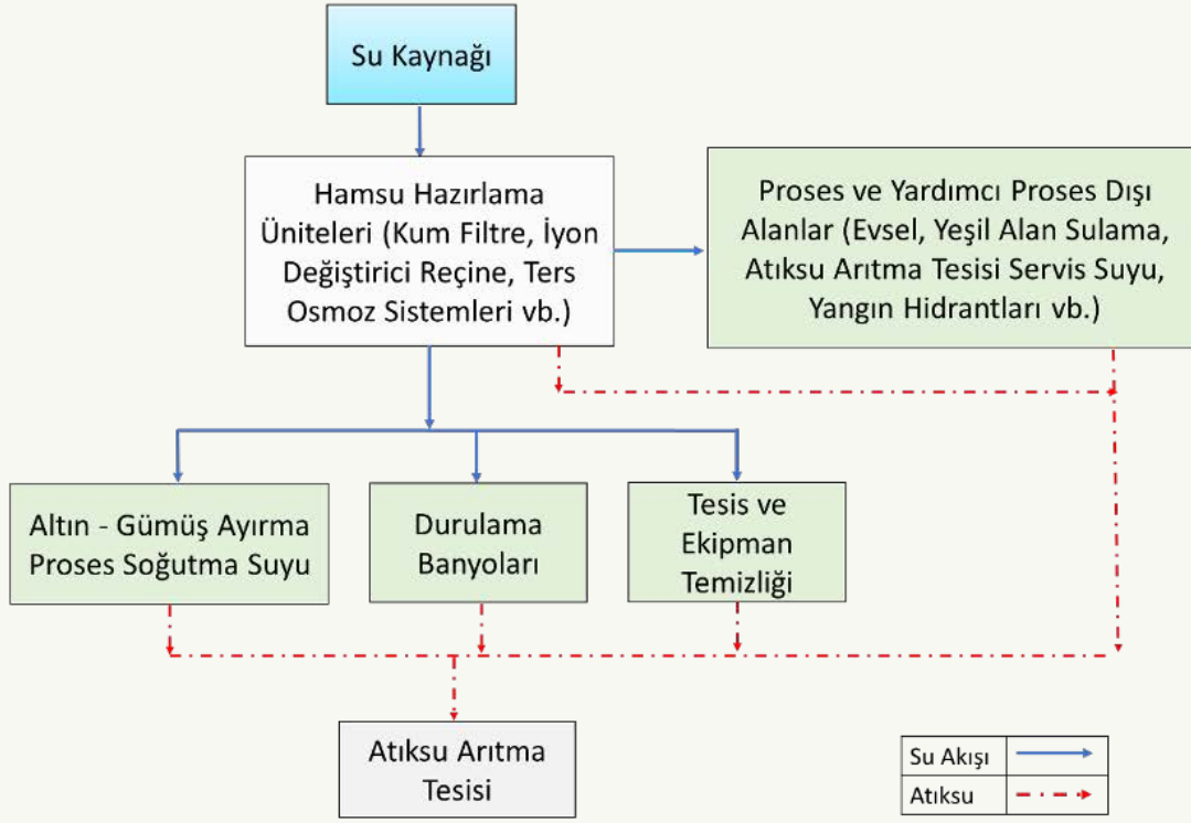
Değerli Metal Üretimi Sektörü Su Akım Şeması
