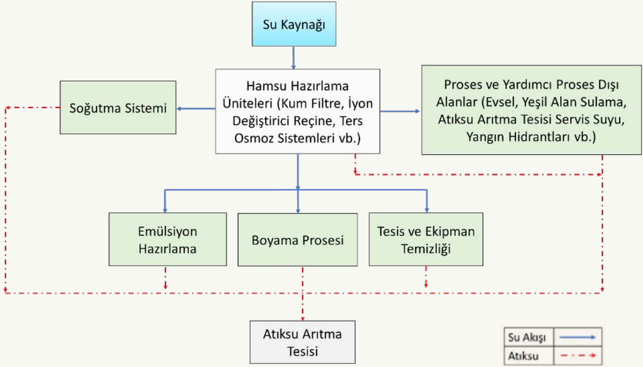
Barların Soğuk Çekilmesi Sektörü Su Akım Şeması
