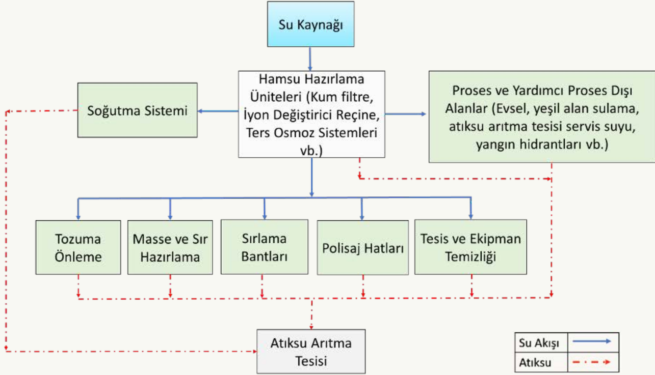
Seramik Karo ve Kaldırım Taşları İmalatı Sektörü Su Akım Şeması
