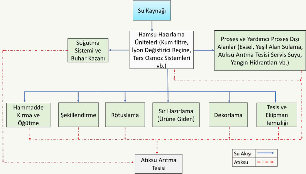
Seramik Ev ve Süs Eşyaları İmalatı Sektörü Su Akım Şeması
