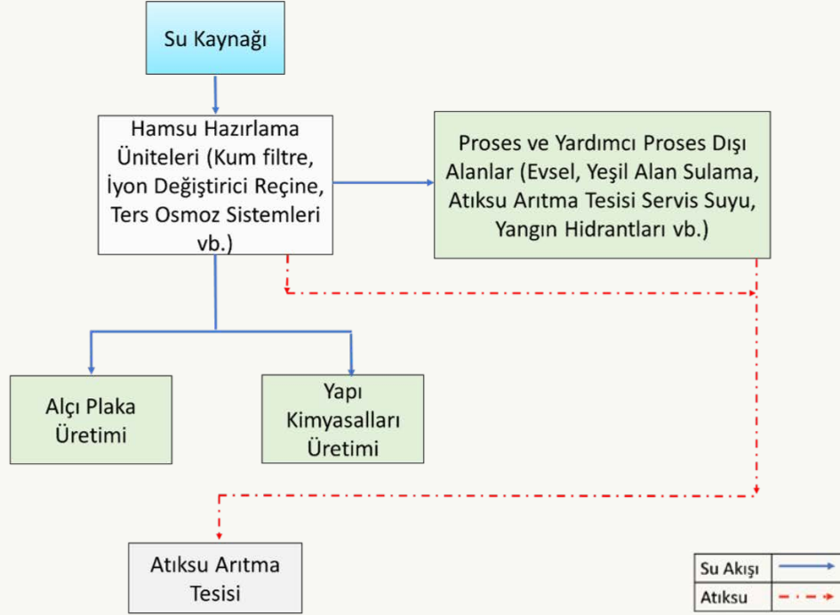
İnşaat Amaçlı Alçı Ürünlerinin İmalatı Sektörü Su Akım Şeması
