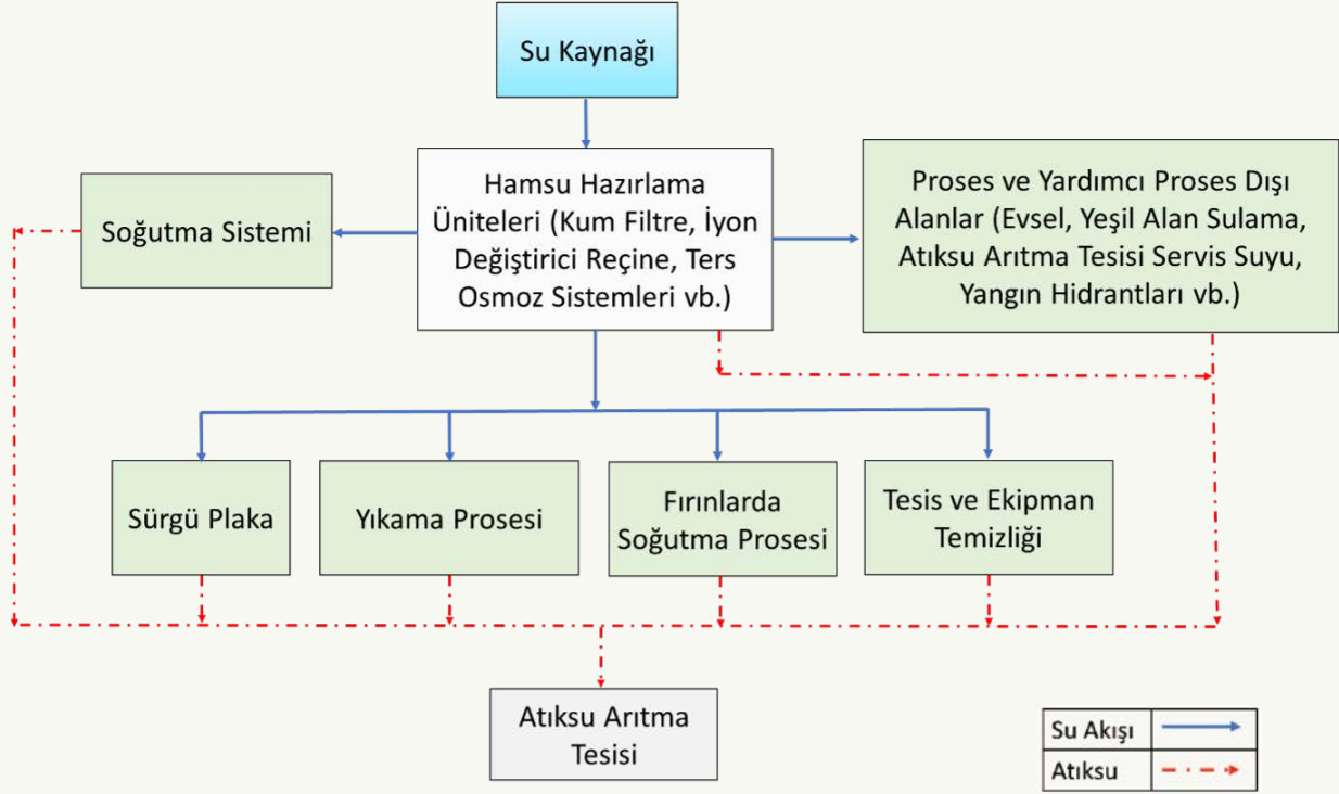
Ateşe Dayanıklı (Refrakter) Ürünlerin İmalatı Sektörü Su Akım Şeması
