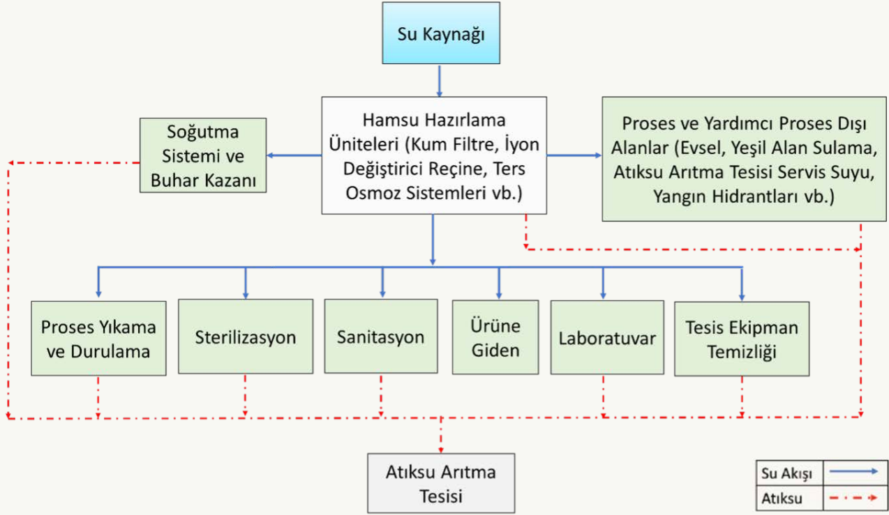
Eczacılaşa İlişkin İlaçların İmalatı Sektöründe Su Akım Şeması
