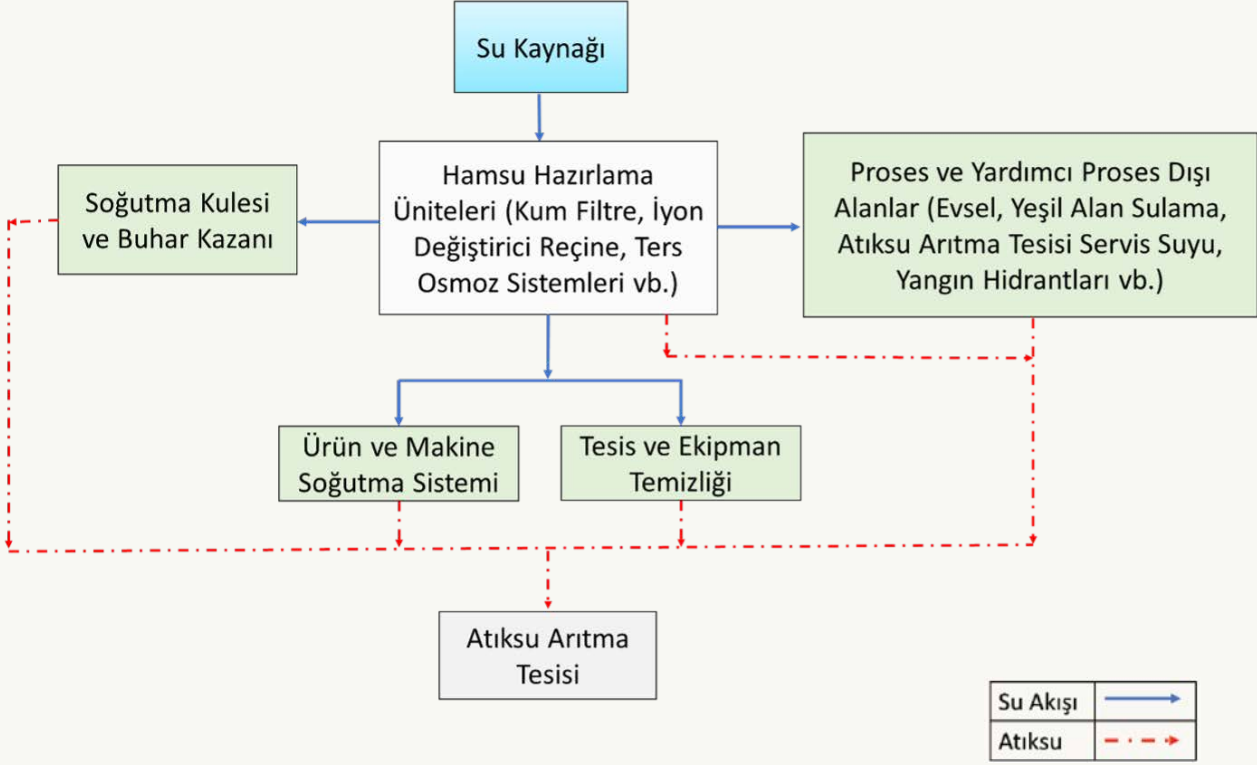
Sanayi Gazları İmalatı Sektörü Su Akım Şeması
