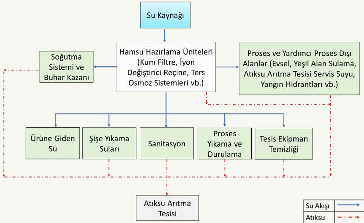
Parfümlerin, Kozmetiklerin ve Kişisel Bakım Ürünlerinin İmalatı Sektörü Su Akım Şeması
