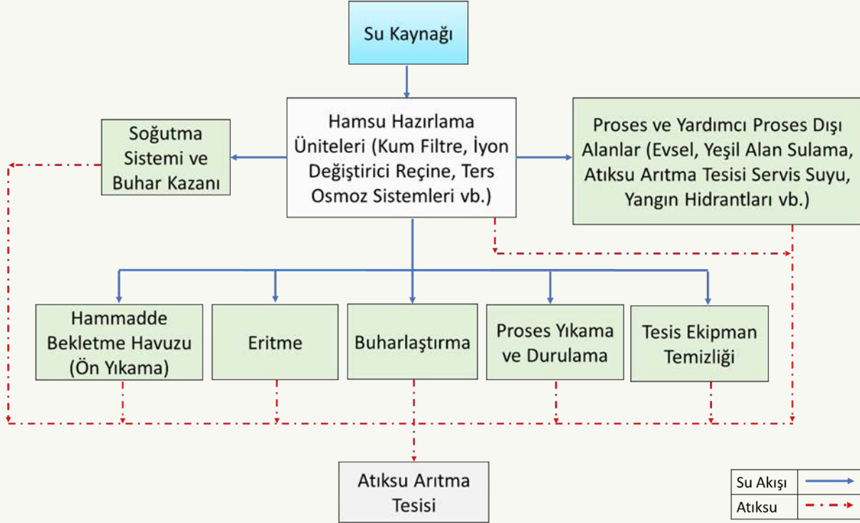
Başka Yerde Sınıflandırılmamış Diğer Kimyasal Ürünlerin İmalatı Sektörü Su Akım Şeması
