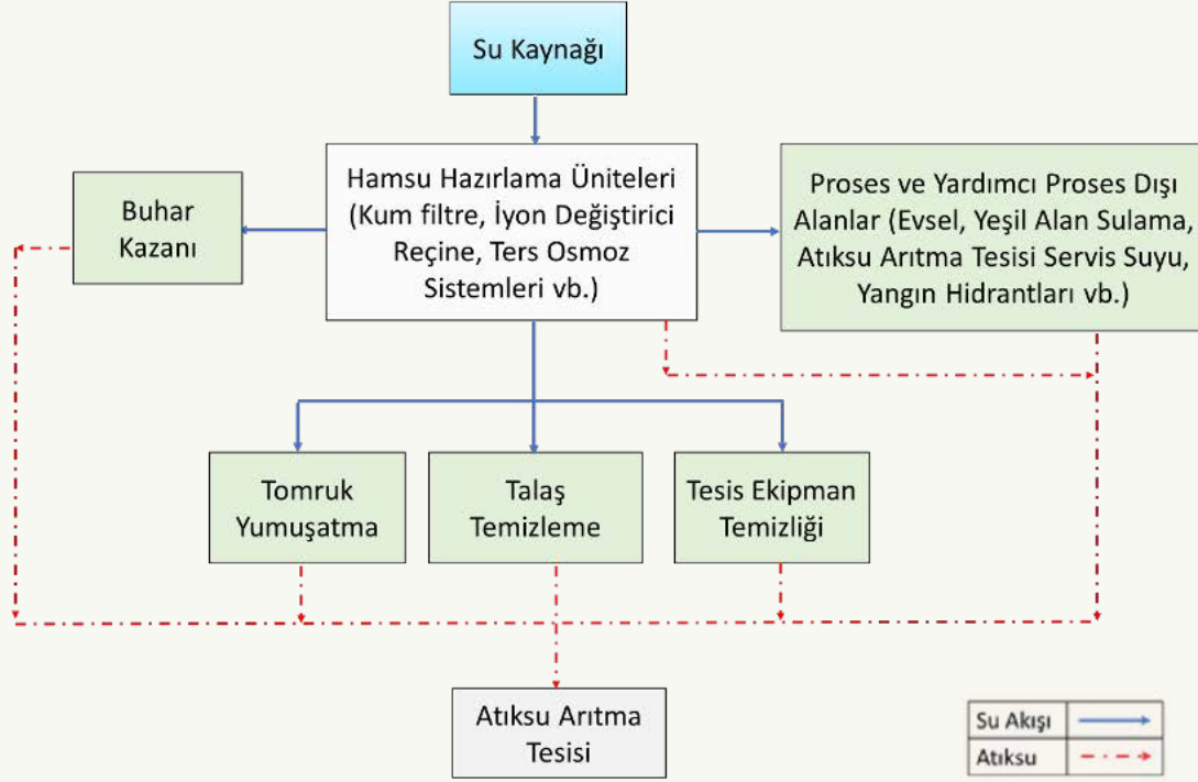
Diğer Ağaç Ürünleri İmalatı; Mantardan, Saz, Saman vb. Örme Malzemelerinden Yapılmış Ürünlerin İmalatı Sektörü Su Akım Şeması
