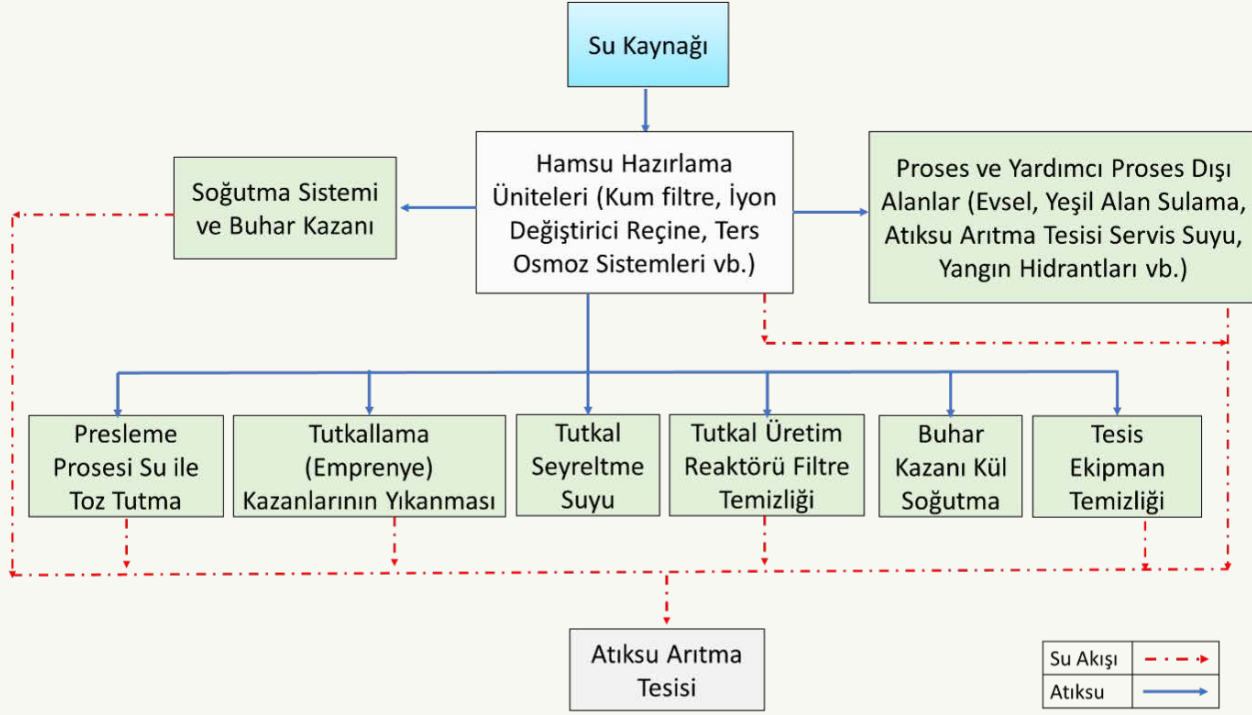
Ahşap Kaplama Paneli ve Ağaç Esaslı Panel İmalatı Su Akım Şeması
