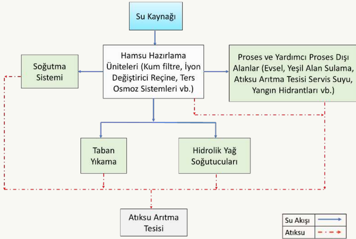
Ayakkabı, Bot, Terlik vb. İmalatı Sektörü Su Akım Şeması
