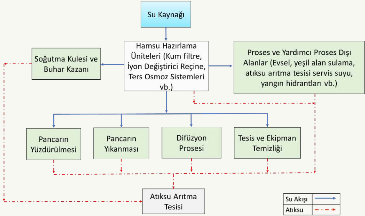
Şeker İmalatı Sektörü Su Akım Şeması
