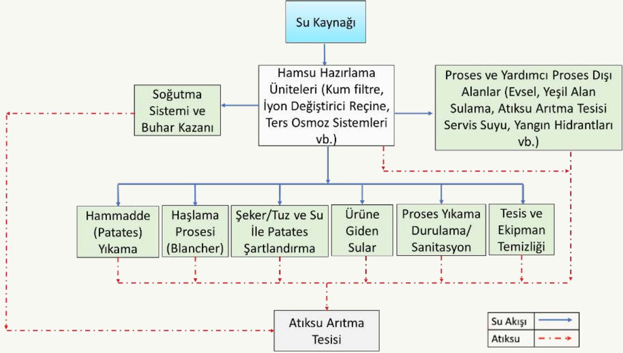
Patatesin İşlenmesi ve Saklanması Sektörü Su Akım Şeması
