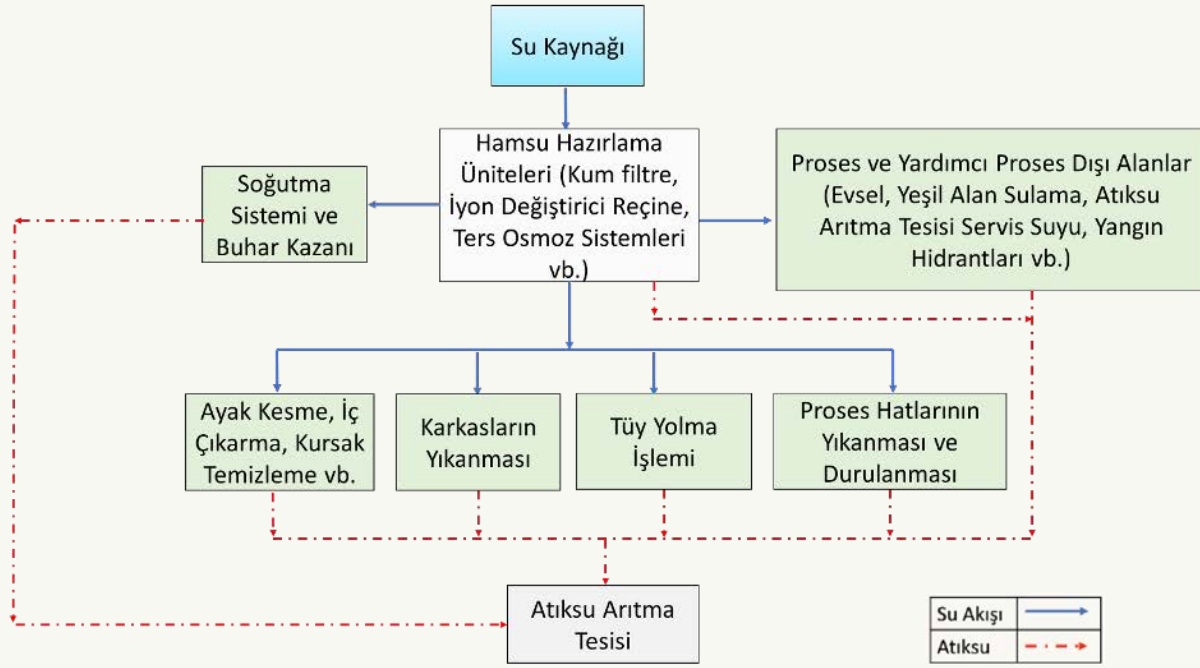
Kümes Hayvanları Etlerinin İşlenmesi Ve Saklanması Sektörü Su Akım Şeması
