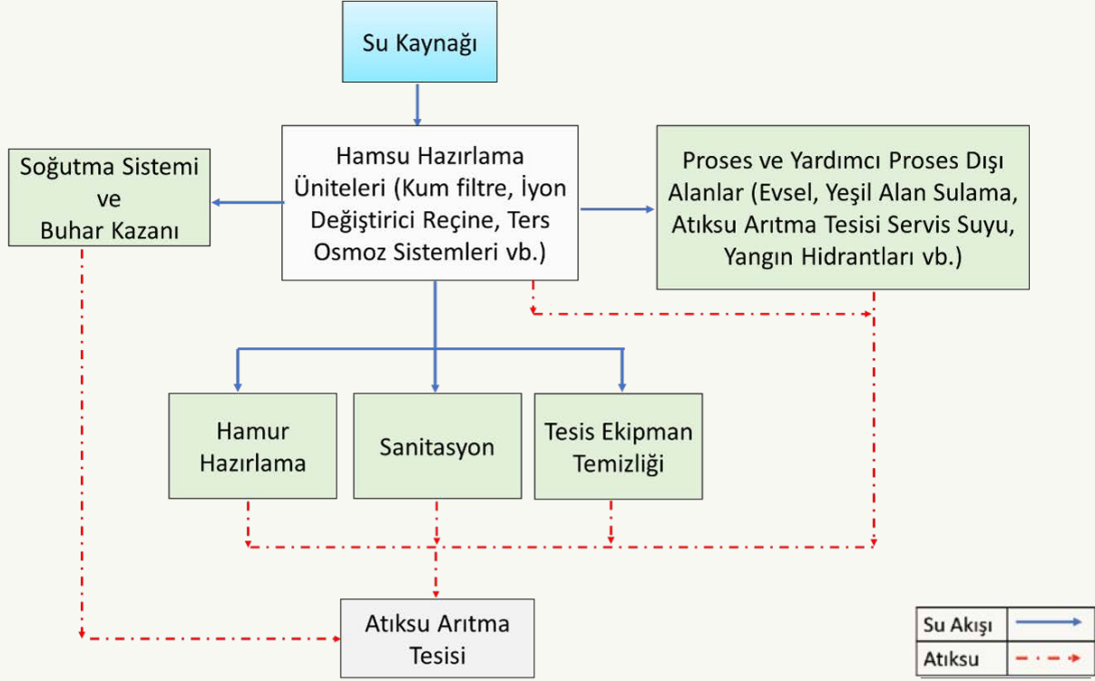
Ekmek, Taze Pastane Ürünleri ve Taze Kek İmalatı Sektörü Su Akım Şeması
