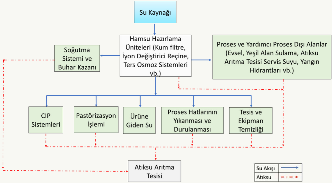
Dondurma İmalatı Sektörü Su Akım Şeması
