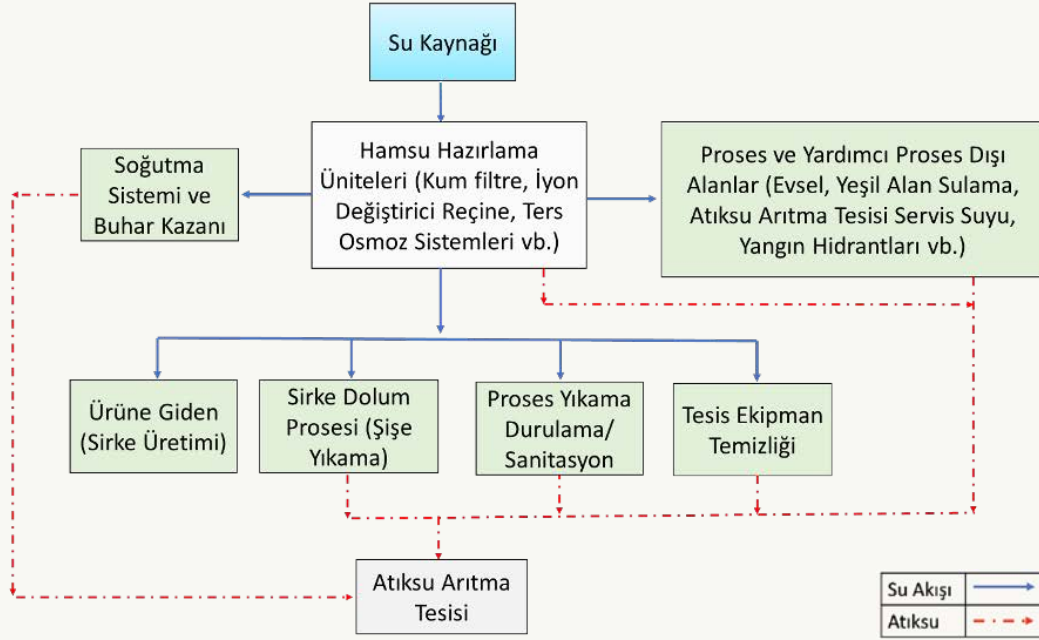
Baharat, Sos, Sirke ve Diğer Çeşni Maddelerinin İmalatı Sektörü Su Akım Şeması
