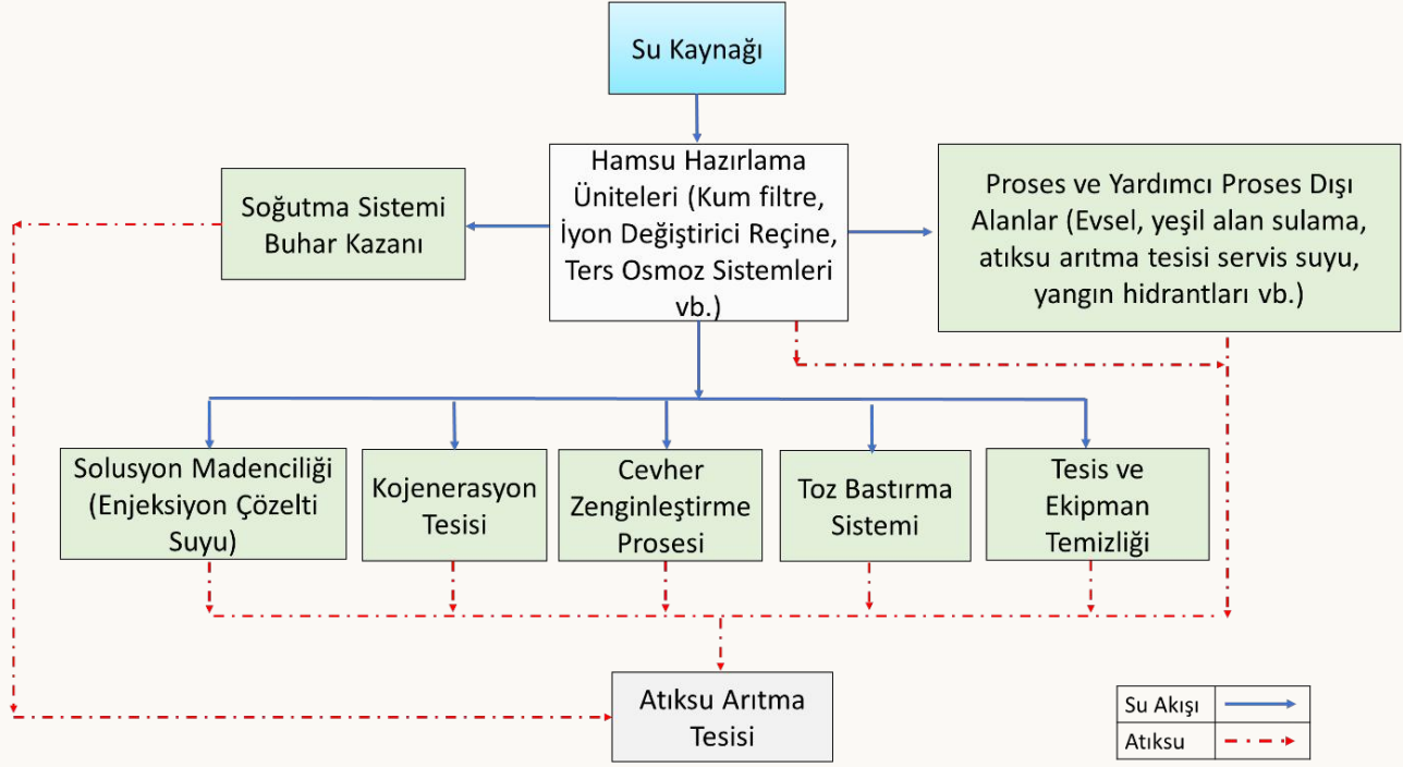
Kimyasal ve Gübreleme Amaçlı Mineral Madenciliği Sektörü Su Akım Şeması
