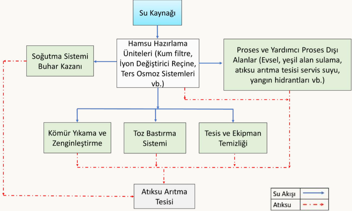
Taş Kömürü Madenciliği Sektörü Su Akım Şeması
