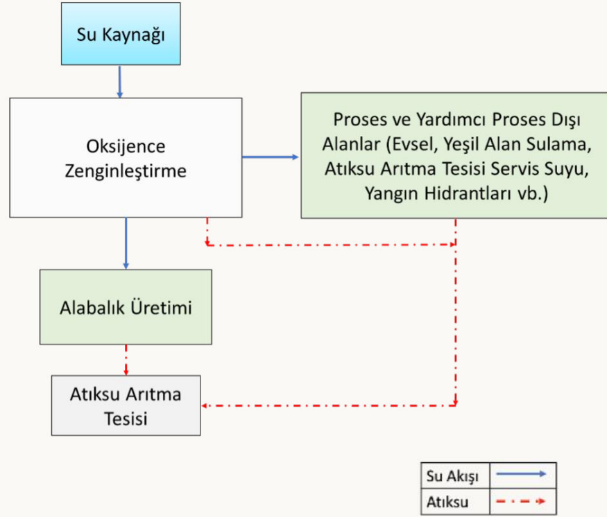
Tatlı Su Balıkçılığı Sektörü Su Akım Şeması
