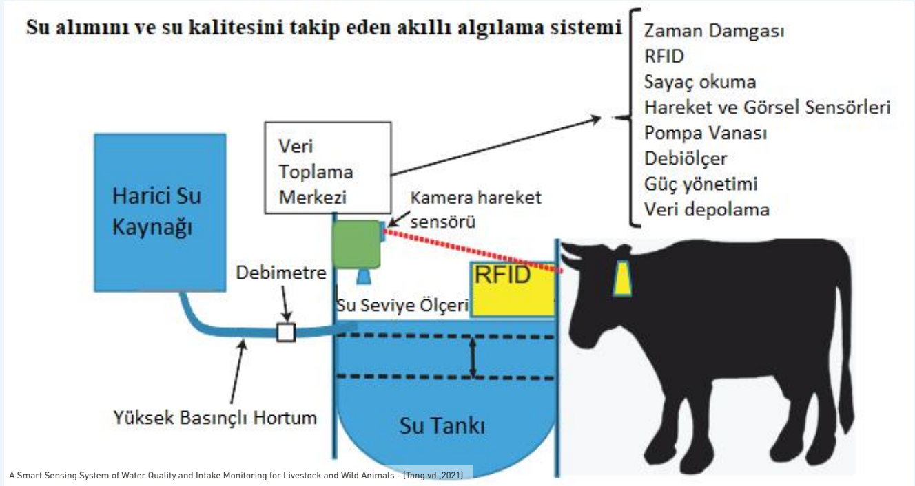
Çiftlik Hayvanları İçin Su Kalitesi ve Su Alımını İzlemeye Yönelik Akıllı Algılama Sistemi
