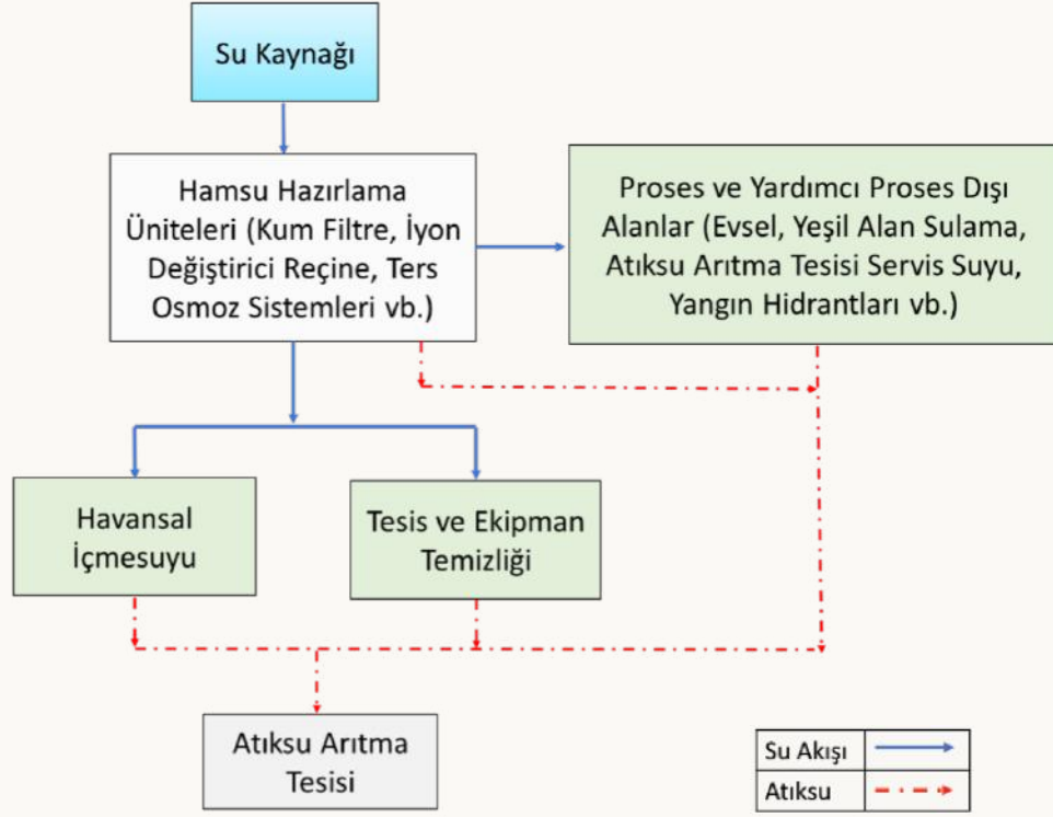
Diğer Sığır ve Manda Yetiştiriciliği Sektörü Su Akım Şeması
